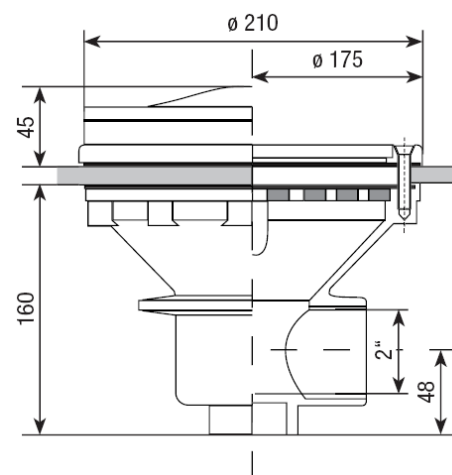
Aufbau Bodenplatte und Montage Bodenablauf
